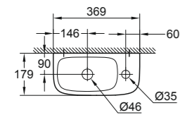
39 327 000 39 327 00H* Mini handrinse basin 37 cm
