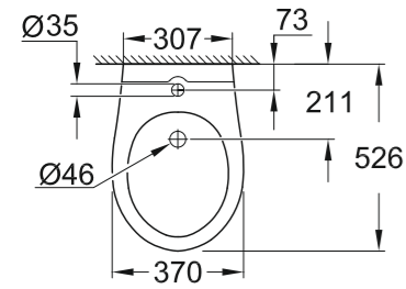
39 433 000 Wall hung bidet
