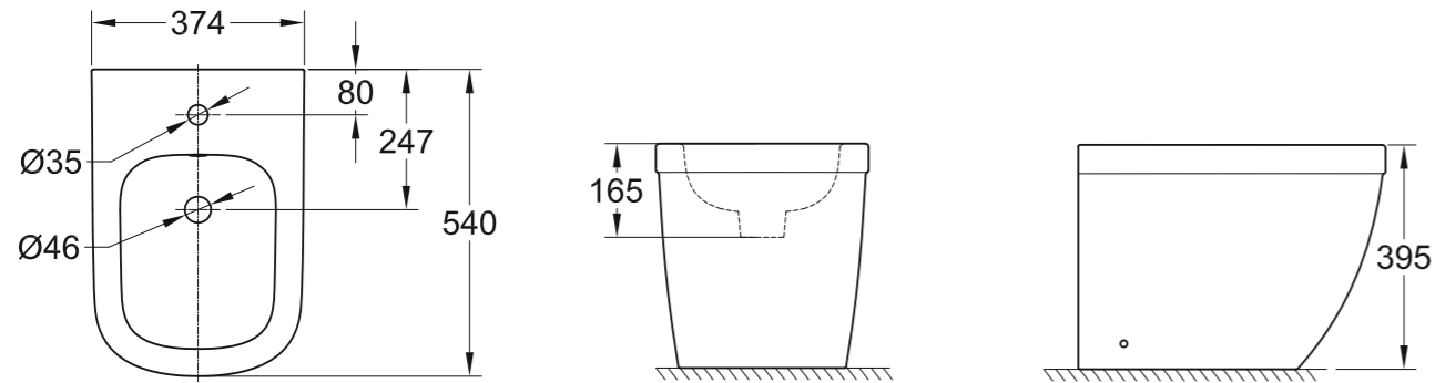
39 340 000 39 340 00H* Floorstanding bidet
